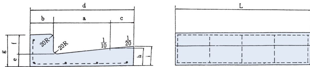
鉄筋コンクリートL形
