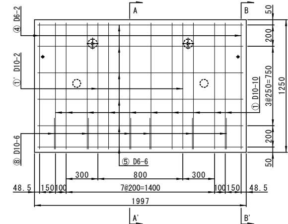
配筋図(縦壁)
