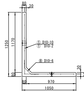
配筋図(側面A-A')
