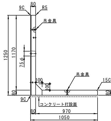
側面図
