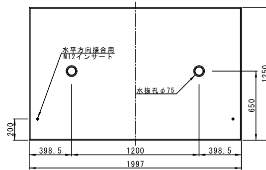
正面図
