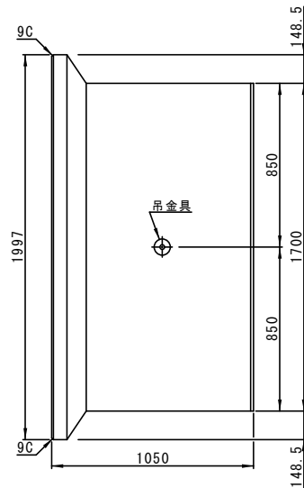
平面図
