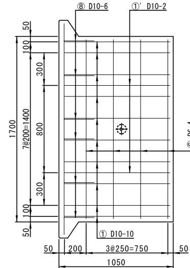
配筋図(底版)
