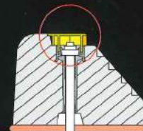
現状仕様キャップ断面図
