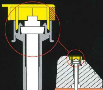
ホルダー断面図
